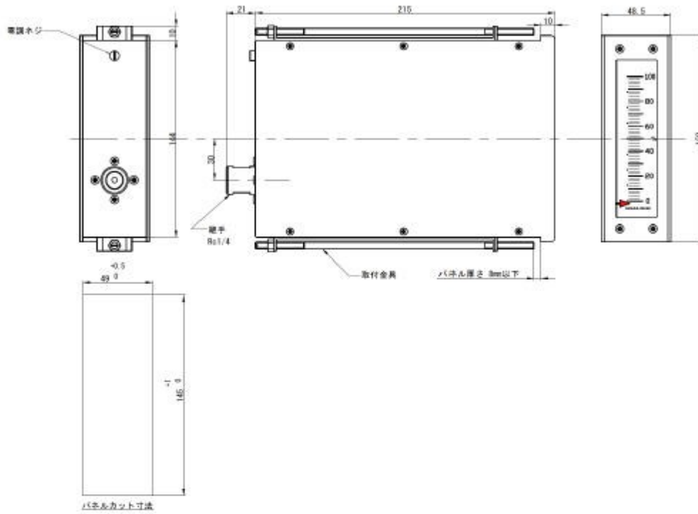
外形図
