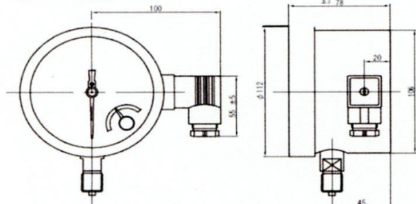
CGM-100-A 1接点
