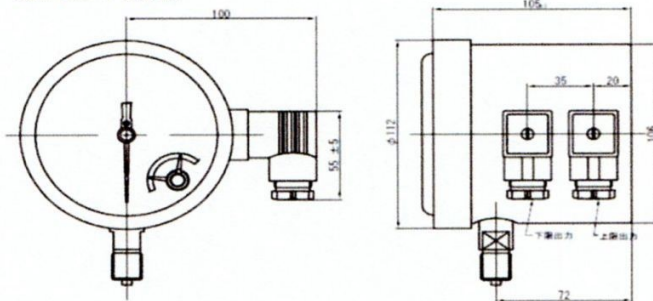
CGM-100-A 2接点
