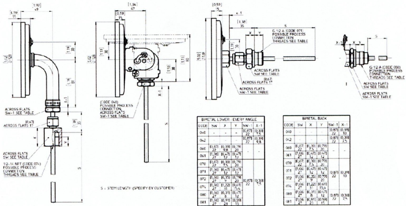
E型 外形図 単位:mm (inch)
