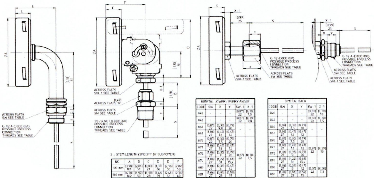
A型 外形図 単位:mm (inch)
